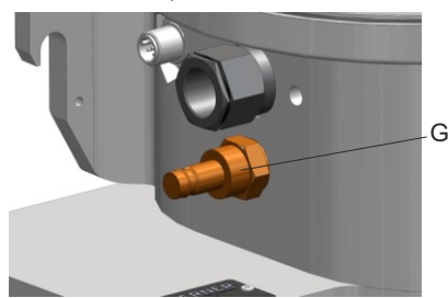
Raccord de remplissage "G" Obturbateur de protection
