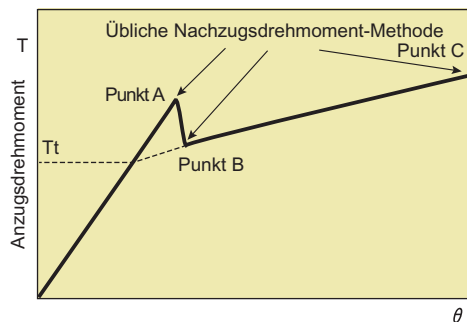
Abbildung-1 Übliche Nachzugsdrehmoment-Methode
