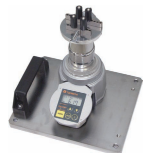
BTGE-G mit Tischbefestigung und Messstand
