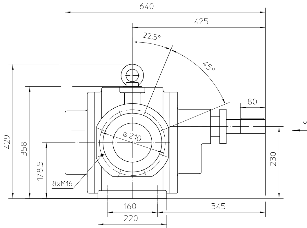
Ansicht Y
