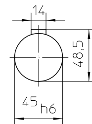
Ansicht Y
