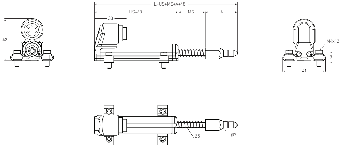
CN5B: M16, 5 pin konnektör çıkışlı (opsiyonel)
