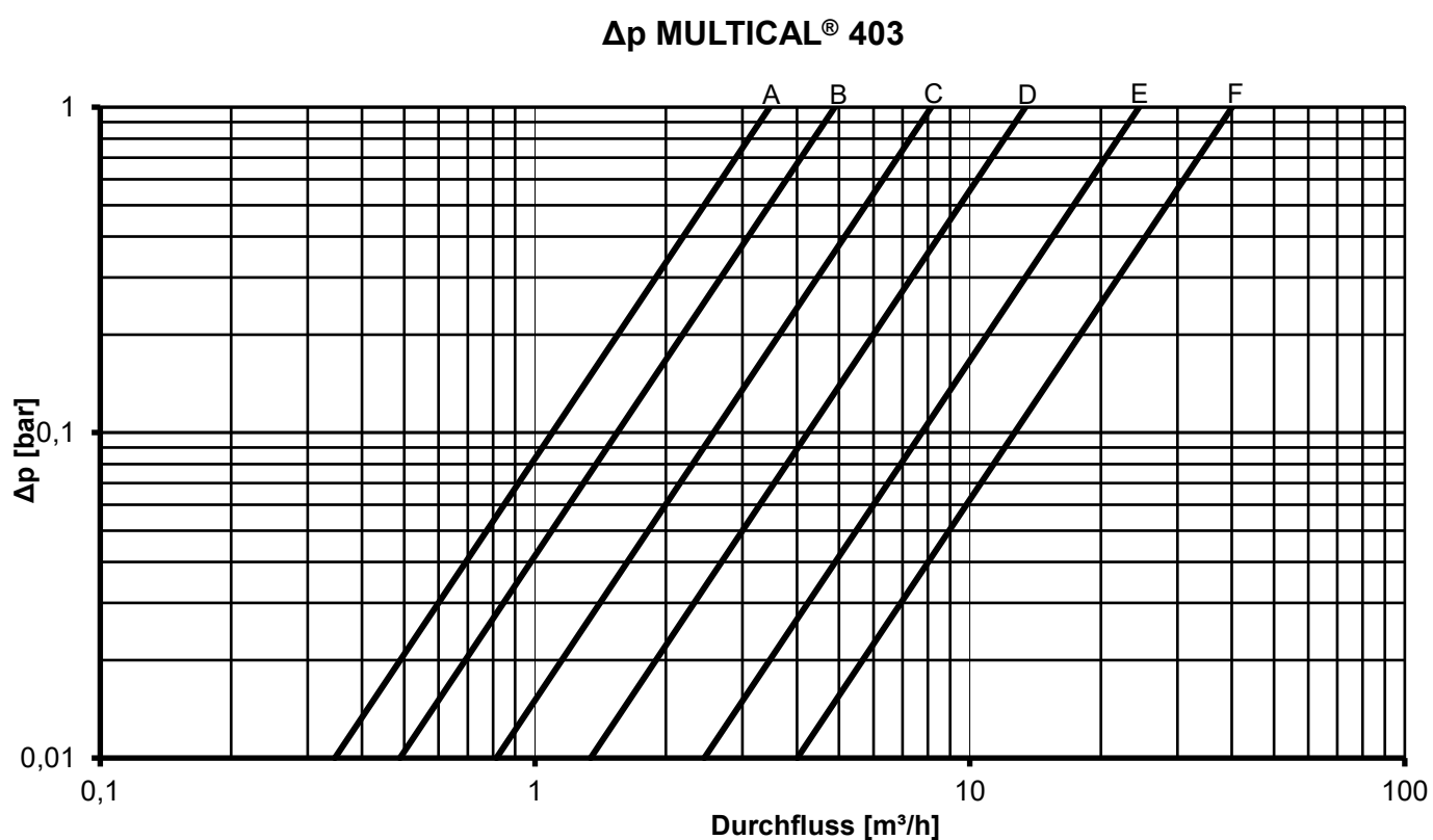
Diagramm 3: Druckverlustkurven
