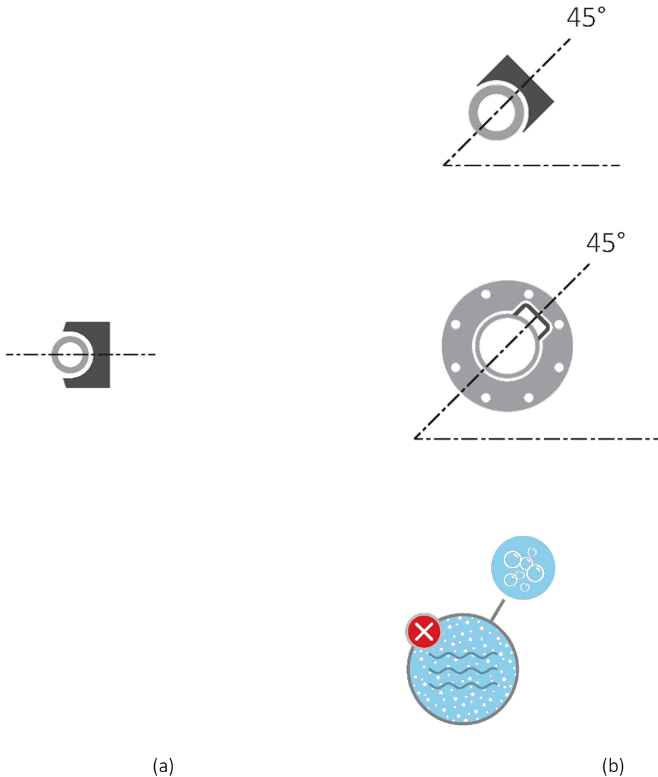
Abb. 5. Empfohlene Orientierung der Kamstrup-Durchflusssensoren um die Rohrachse bei waagerechter Montage für Kälte- und kombinierte Wärme-/Kälteinstallationen. (a) Zählergehäuse mit Gewinde mit q_p \leq 2,5 \text{ m}^3/\text{h} . (b) Zählergehäuse mit Gewinde mit q_p \geq 3,5 \text{ m}^3/\text{h} und Zähler mit Flansch.
