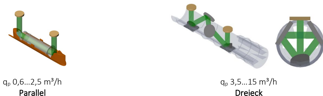
Abb. 13: Signalwege im MULTICAL® 403. Ultraschallsignale werden von den Ultraschallwandlern abhängig von der Konstruktion über 2 oder 4 Reflektoren gesendet. Für kleine Zähler ( q_p 0,6...2,5 m³/h) ist ein paralleler Schallweg hinreichend. Zur Erfassung der Durchflussänderungen entlang des Rohrdurchmessers (das Durchflussprofil) im Durchflusssensor wird in größeren Zählern ( q_p 3,5...15 m³/h) ein dreieckiger Schallweg verwendet. In beiden Konstruktionen verändern sich die Laufzeiten für das Signal in Richtung des Durchflusses und entgegen dem Durchfluss.
