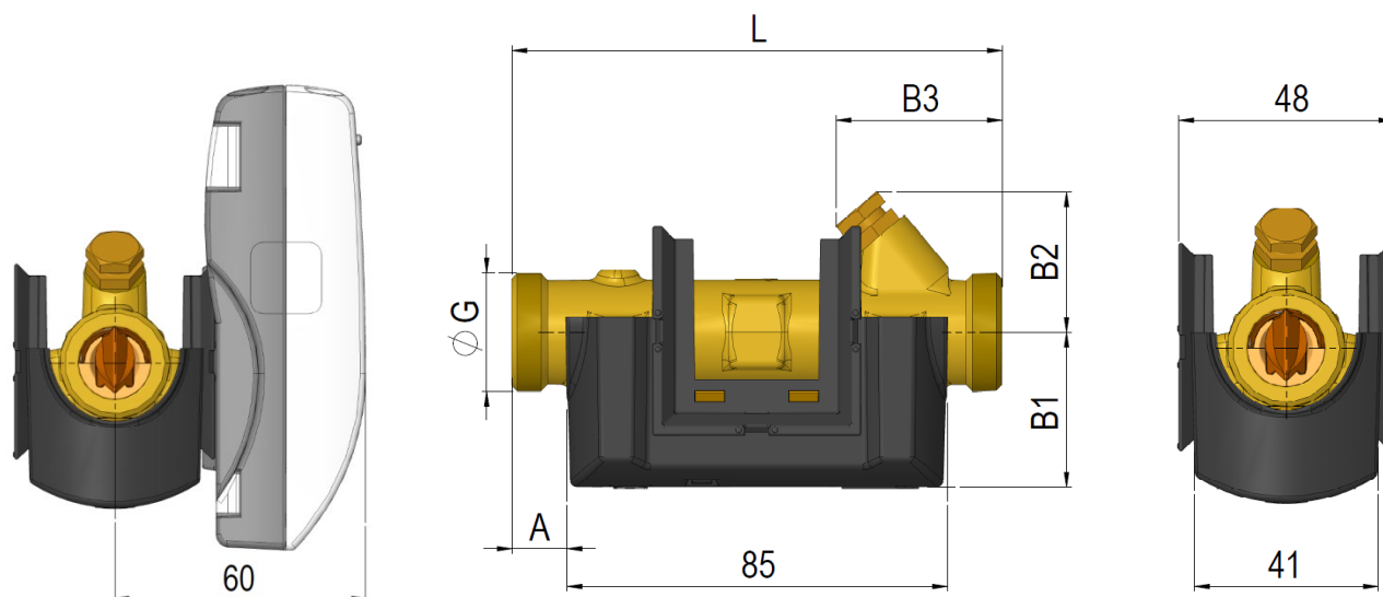
Abb. 10: Durchflusssensor mit G \frac{3}{4} und G1 Gewindeanschluss
