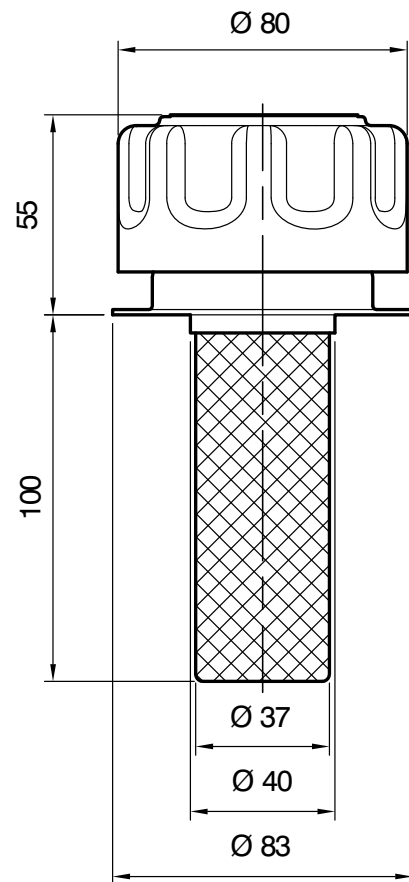
Einschweißflansch Weld flange
