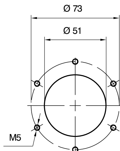
Befestigungsflansch Mounting flange
