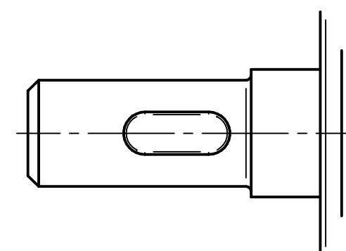
Passfeder / Key DIN 6885 - A4x4x10
