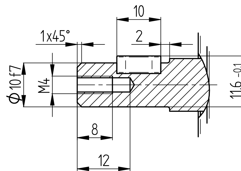
Passfeder / Key DIN 6885 - A4x4x10
